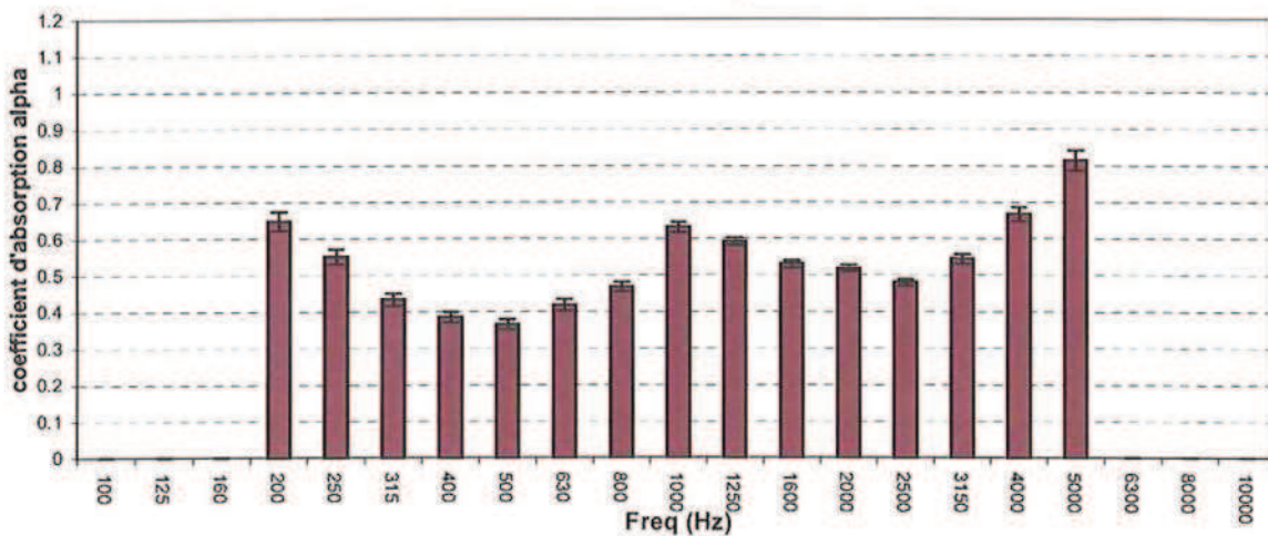
Niveaux d'absorption
